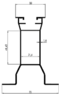
10 cm Profile 1795 1446 gr/m
