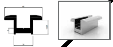
Mid Clamp 694 731 gr/m
