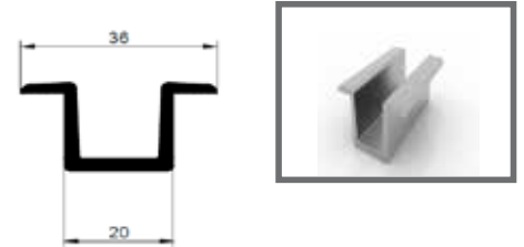
Mid Clamp 1136 456 gr/m
