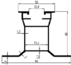
6 cm Profile 1796 1063 gr/m
