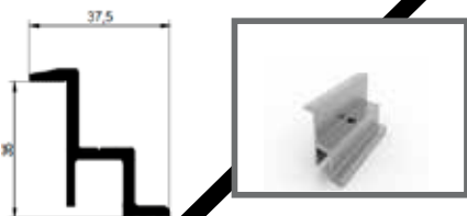
35'lik H End 1624 634 gr/m
