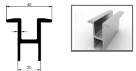
H Mid 1623 772 gr/m
