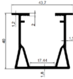
Bottom Rail 1809 714 gr/m
