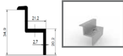
35'lik End Clamp 1134 461 gr/m
